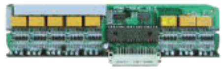
Card CE8 Card 8 máy lẻ nội bộ
